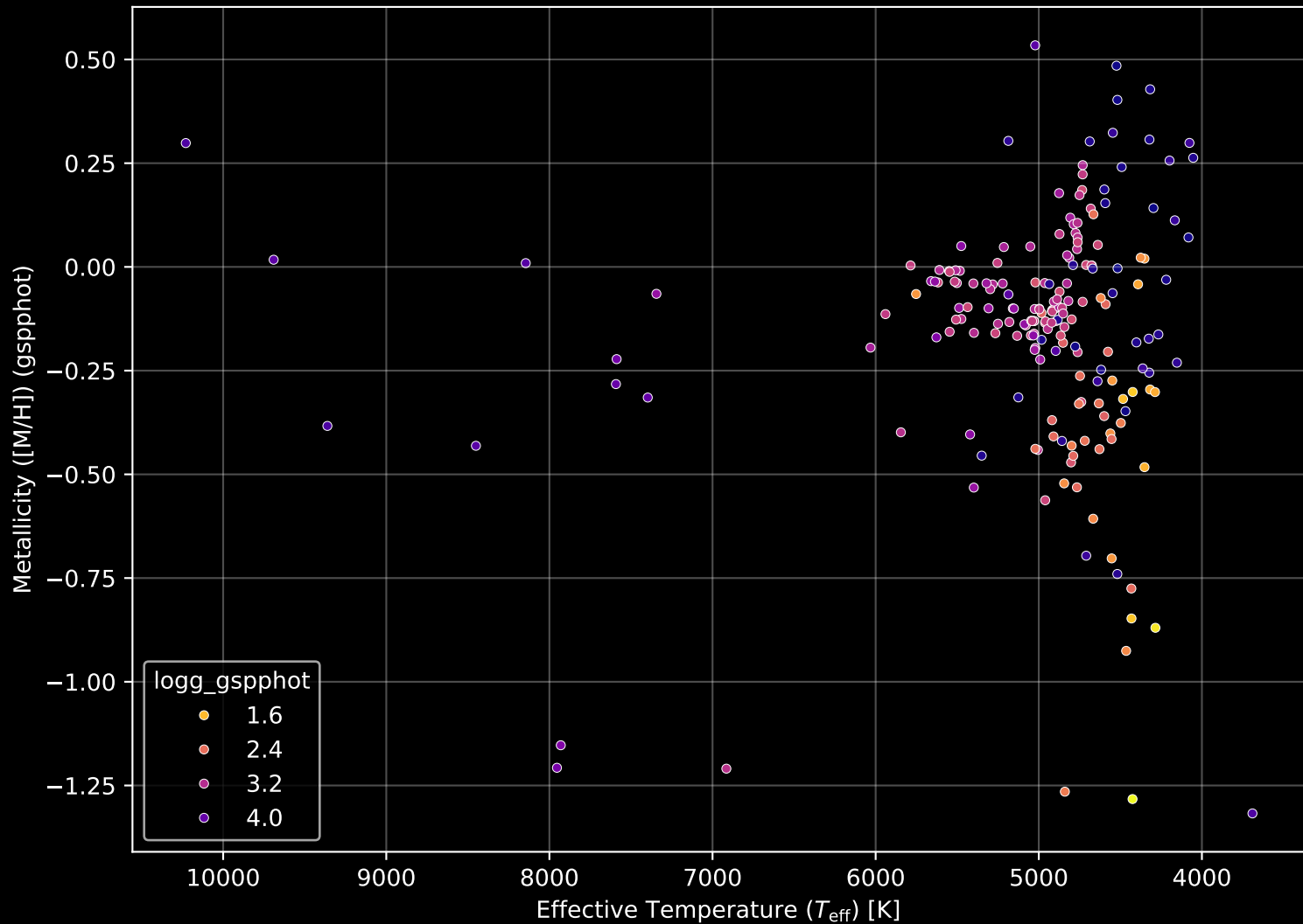
APOGEE DR17 Field: [020-16] Stellar Population Parameters (n= 197)
